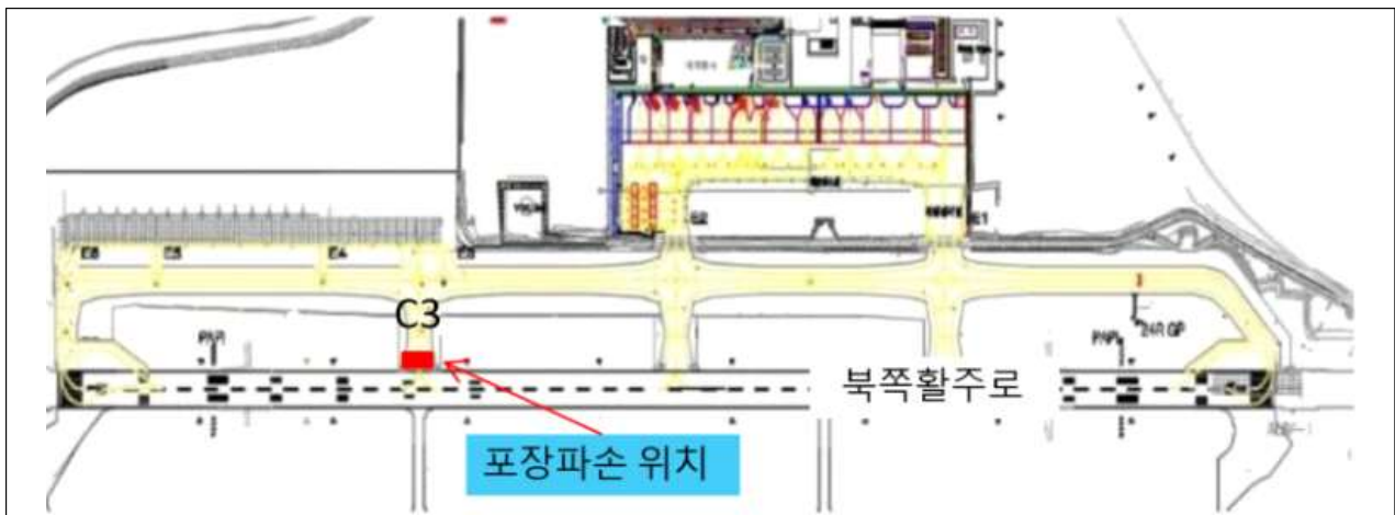
【그림】 ☆☆공항 C3 유도로 및 포장파손 위치
