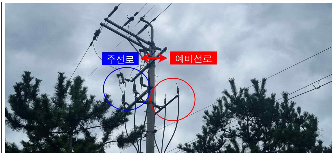
【그림2】한전인입전주 현황
